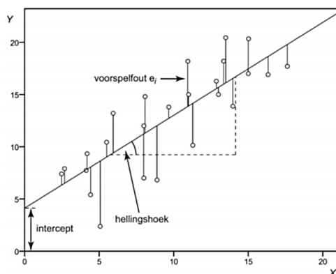
Figuur 1. Voorspelfouten ( e_i = Y - \hat{Y}_i ) bij een lineair regressiemodel
